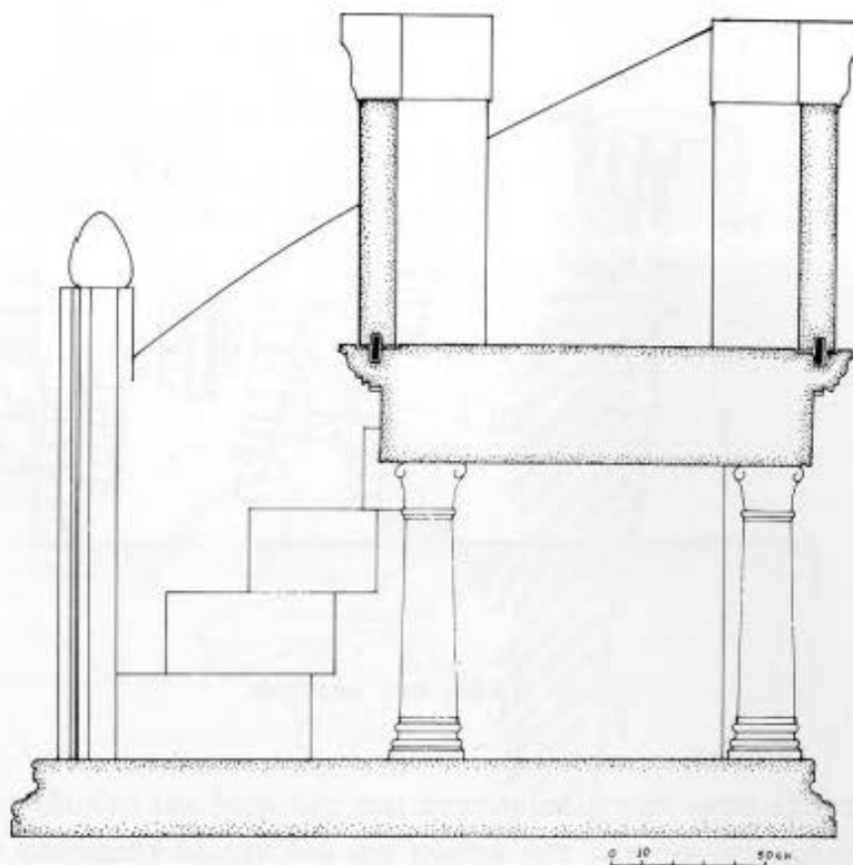
Σχ. 2. Ριπιδόσχημος άμβωνας - Τομή.
