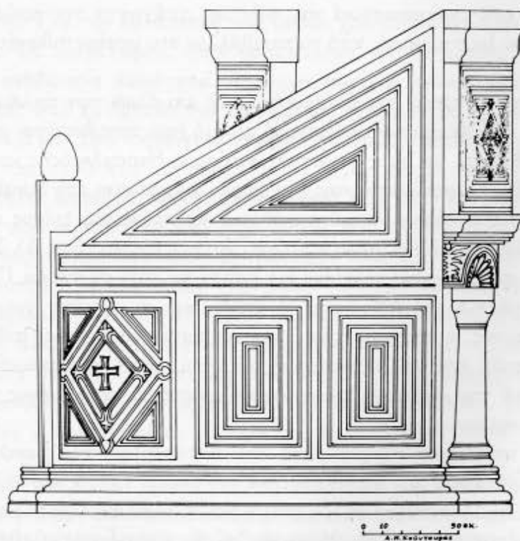
Σχ. 3. Ριπιδόσχημος άμβωνας - Πλάγια όψη.
