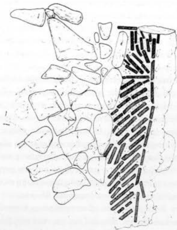
Σχ. 5. Επιτύμβιο σήμα.
