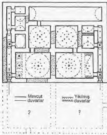
Demirhisar'daki XVI. yüzyıla ait çifte hamamın planı (M. Kiel arşivi)
