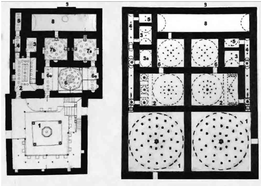
Εικ. 43. Αριστερά: Αποτύπωση του μονού Χαμάμ της Αγοράς στο Elbasan (Πηγή: Roberto B.F. Castiglia και Marco Giorgio Bevilacqua, ό. π., σ. 310) - Δεξιά: Αποτύπωση του αντίστοιχου διπλού χαμάμ του Σιδηροκάστρου (Πηγή: Michael Kiel, "Demirhisar", ό. π., σ. 152) - Υπόμνημα: 1. Χώρος Εισόδου/ Αποδυτηρίων (camekân), 2. Χλιαρό τμήμα (soğukluk), 3. Χώρος καθαρισμού/ πλυσίματος και στεγνώματος πετσετών, 3a. Ατομική καμπίνα/μικρό δωμάτιο ανάπαυσης, 4. Και 5. Αποχωρητήρια, 6 και 6a. Ο θερμός χώρος (sicaklik), 7a. και 7b. Χώροι ατμόλουτρων (maghtas ή halvet), 8. Δεξαμενή νερού, 9. Χώρος της Εστίας.
