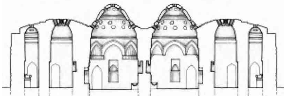
Εικ. 47. Πρόταση αρχιτεκτονικής αποκατάστασης της εγκάρσιας τομής του χαμάμι κατά τον άξονα ανατολής-δύσης, όπου διακρίνονται από αριστερά προς δεξιά: ο πλευρικός διάδρομος του ανδρικού τμήματος, δεξιότερα ο θολωτός χώρος του καθαρισμού/πλυσίματος και στεγνώματος πετσετών και ακόμα δεξιότερα ο κεντρικός θερμός χώρος (sicaklik) που καλύπτεται επίσης από θόλο τύπου Bell dome. Συμμετρικά αναπτύσσονται οι αντίστοιχοι χώροι και στο ανατολικό τμήμα (γυναικείο τμήμα).
