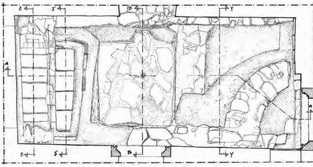
Εικ. 3. Κάτοψη των κτισμάτων που άποκαλύφθηκαν υπό το δάπεδο του νάρθηκος του παρεκκλησίου του Αγίου Νικολάου της Μονής Βατοπεδίου.
