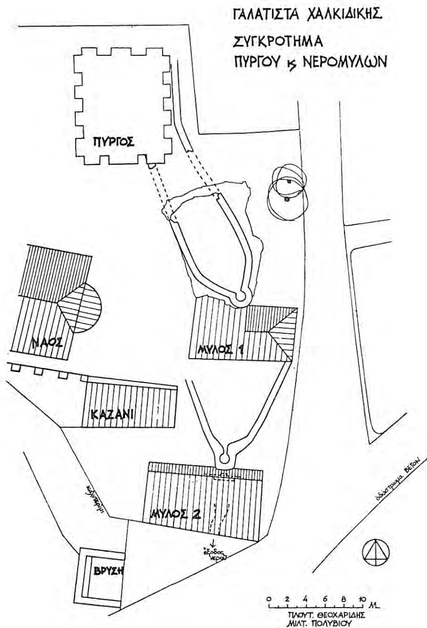
Εικών 20. Σχεδιάγραμμα συγκροτήματος Πύργου και υδρομύλων Γαλατίστης
